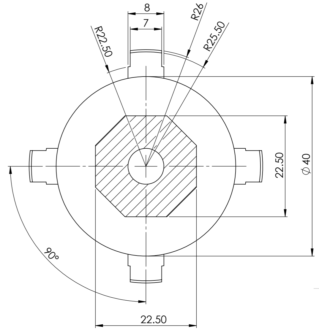
SECTION D-D SCALE 2 : 1
