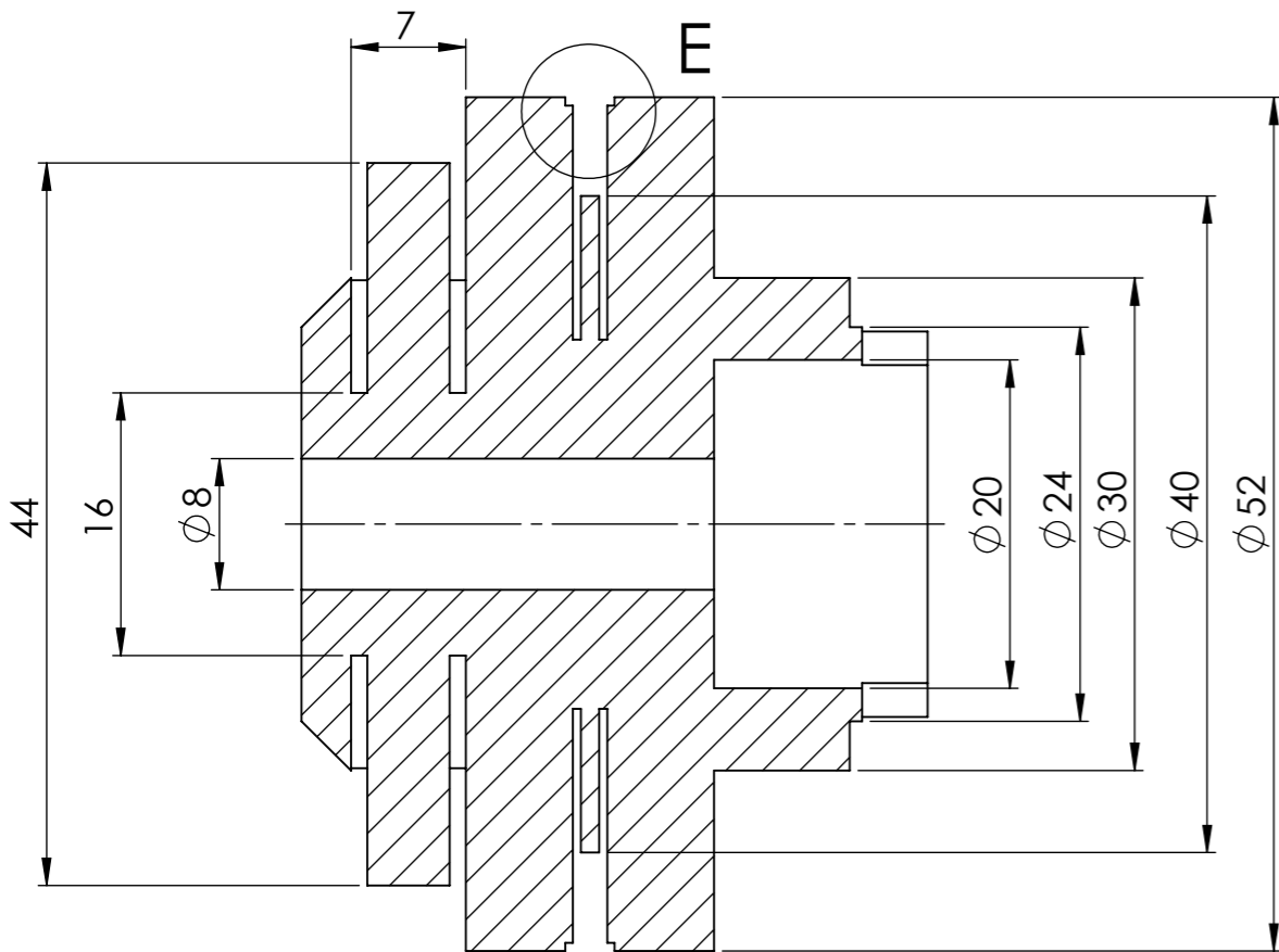
SECTION A-A SCALE 2 : 1
